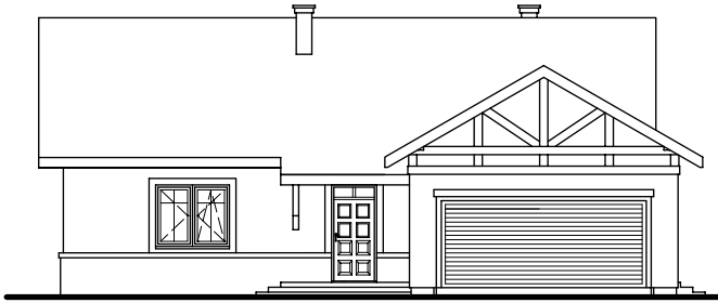
ELEWACJA FRONTOWA
