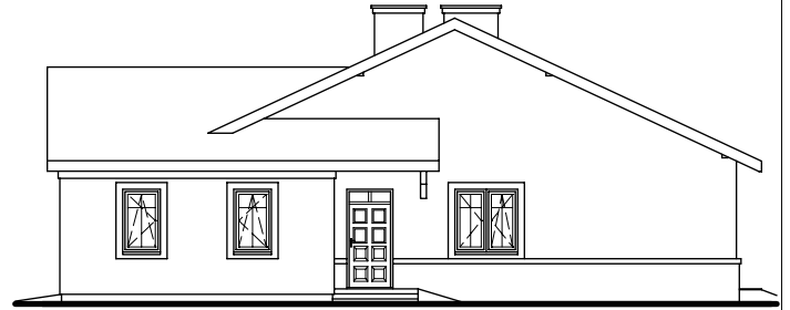
ELEWACJA BOCZNA PRAWA
